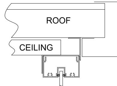
VIEW A-A
